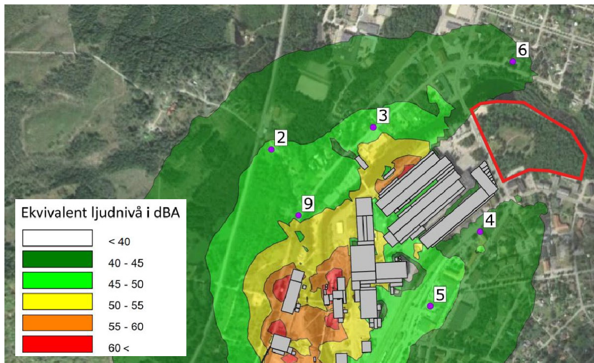
Ekvivalent ljudnivå industribuller.
