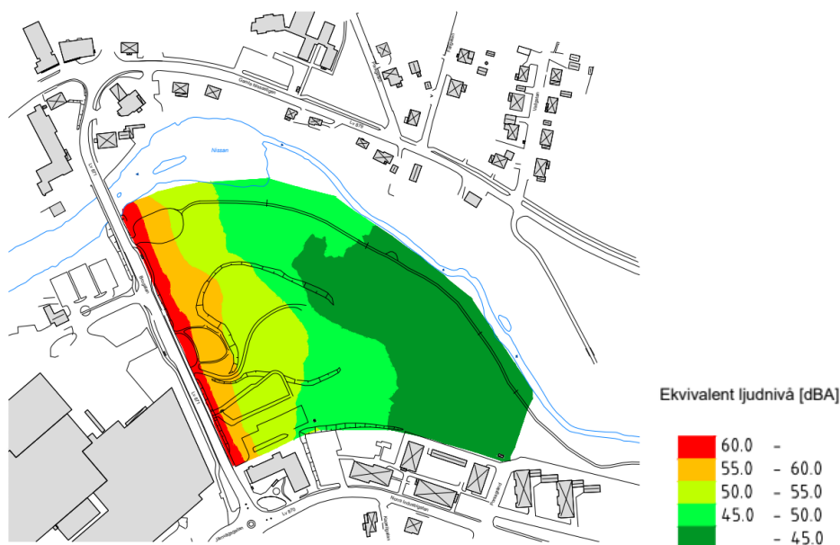
Ekvivalent ljudnivå prognosåret 2040.
