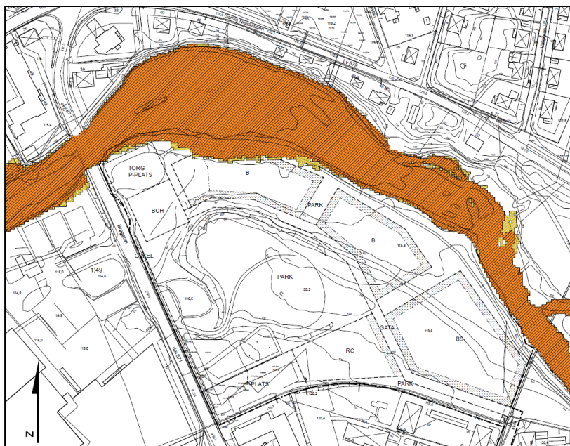
Översvämningskarta. Orange skraffering 100-årsflöde, gul skraffering 200-årsflöde.
